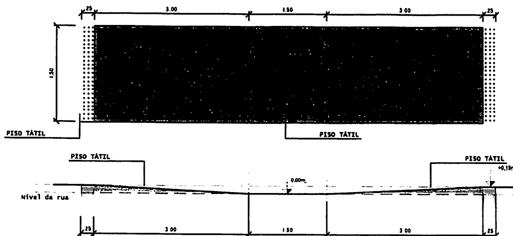
DETALHE - RAMPA ACESSÍVEL Esc. - 1/50
