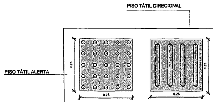
DETALHE - PISO TÁTIL Esc. - S/ escala
