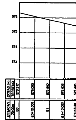
Perfil longitudinal da extensão da Rua Marcondes Balduino
