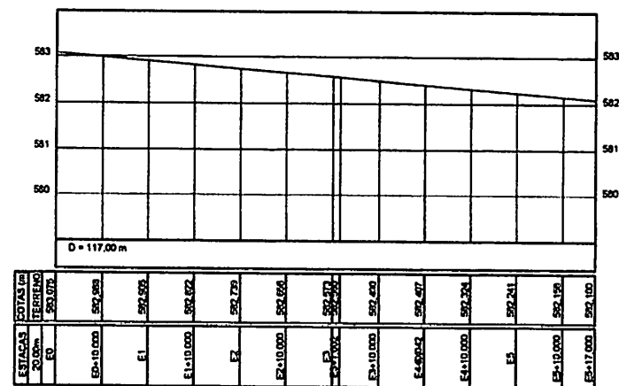
Perfil Longitudinal Rua André Gonçalves
