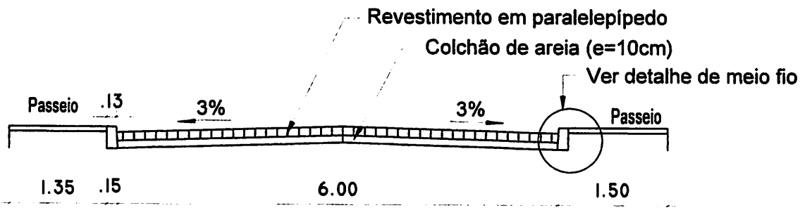
SEÇÃO TRANSVERSAL - TIPO 2 ESCALA - 1/50
