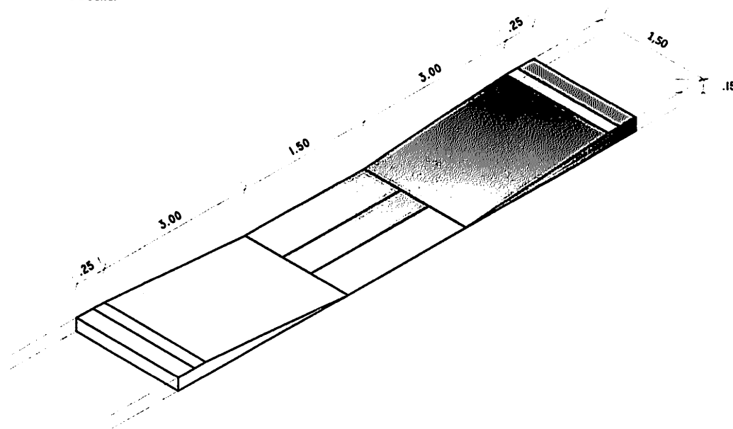
DETALHE ISOMÉTRICO - RAMPA ACESSÍVEL Esc. - S/ escala
