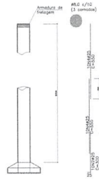
Armação das Pilares (R4) Escala 1:75
