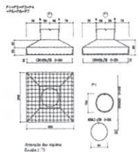
Armação do apoio Escala 1:75
