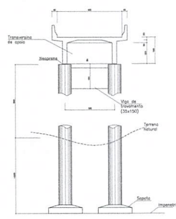
Seção transversal do apoio Escala 1:50
