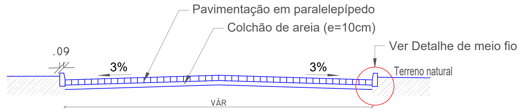
SEÇÃO TRANSVERSAL ESCALA - 1/50
